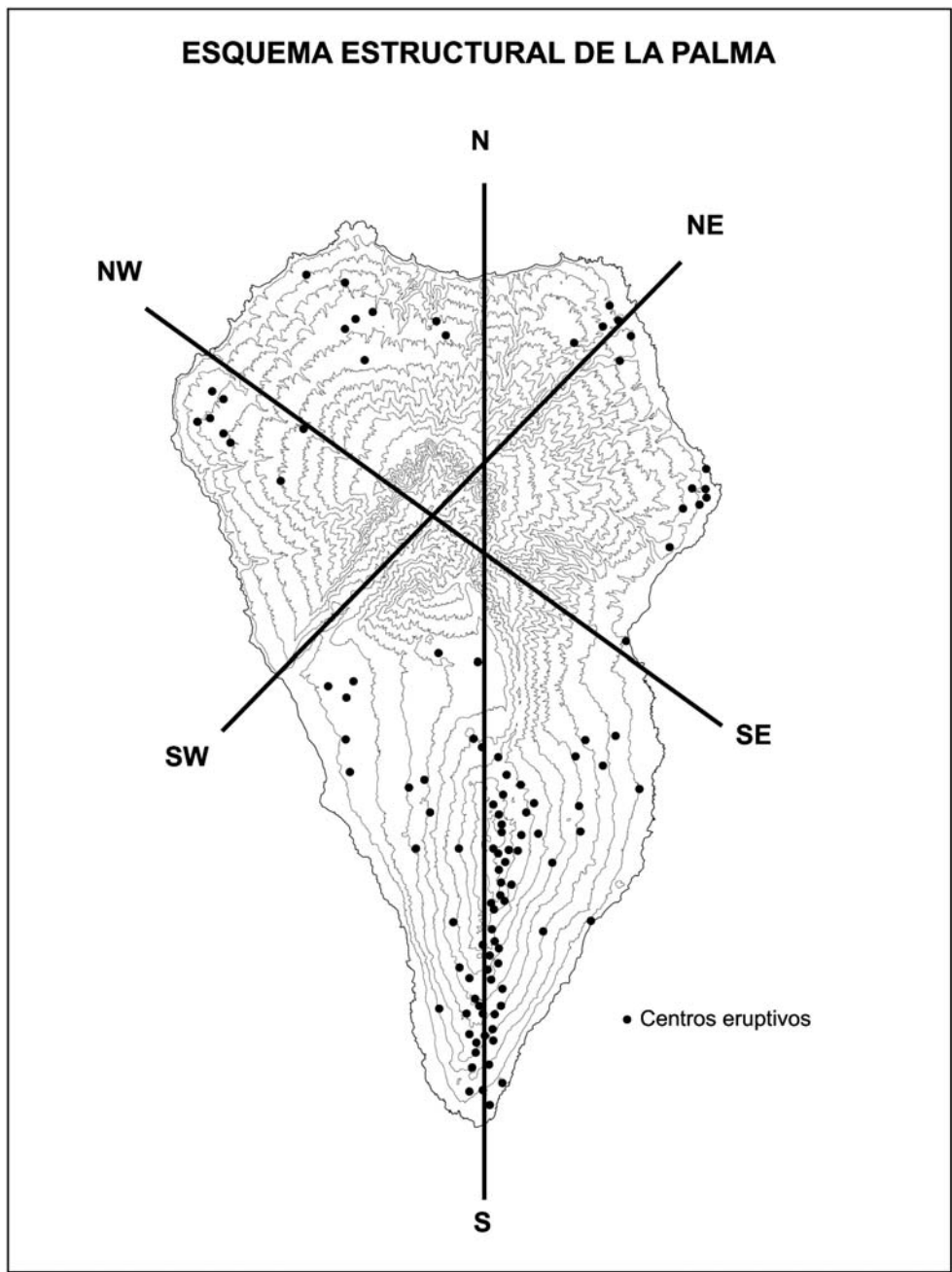
FIG. 2.—Las líneas estructurales, además de organizar los procesos volcánico-constructivos, han sido explotados como líneas de debilidad por los mecanismos erosivos.
